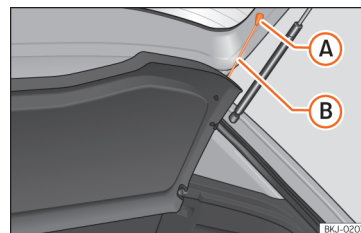
Obř. 116 V zavazadlovém prostoru: demontáž a montáž krytu zavazadlového prostoru.
