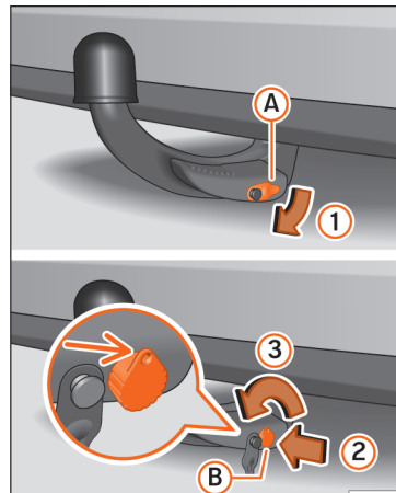
Obr. 175 Demontáž kulové hlavy tažného zařízení
