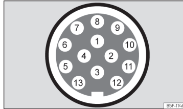
Obr. 168 Schématické zobrazení: Přirazení konektorových kolíků pro napájení přívěsu.
