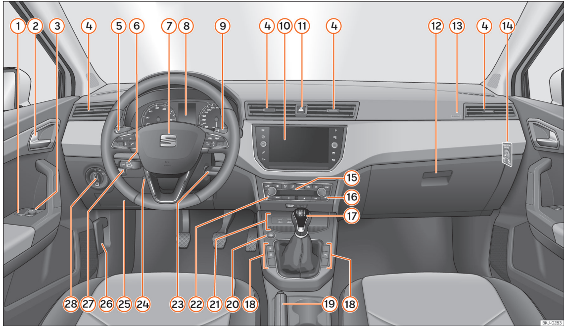
Obr. 64 Prostor řidiče
