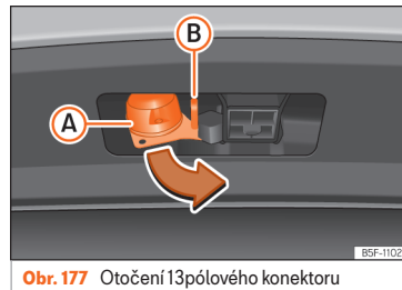
Obr. 177 Otočení 13pólového konektoru
