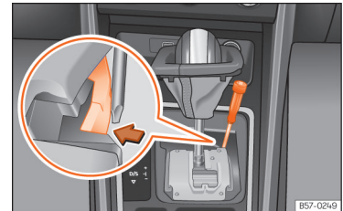
Obr. 144 Volicí páka: Nouzové odblokování z parkovací polohy.
