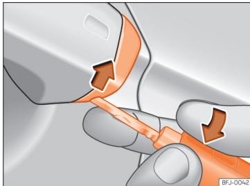
Obr. 90 Klika dveří řidiče: Vypáče krytku.
