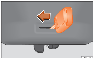
Obr. 94 Detail zavazadlového prostoru: nouzové odemknutí.
