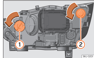
Obr. 55 V motorovém prostoru: žárovka směrového světla ① a žárovka světla DRL (světla pro denní svícení) ②.
