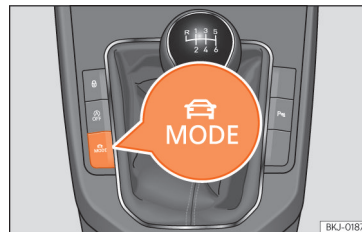
Obr. 145 Vedle řadičové páky: tlačítko MODE .
